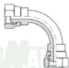
CODO ACCESORIAL 90° HEMBRA LOCA BSP 60° - HEMBRA LOCA BSP 60° RC6032
