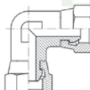
CODO 90° HEMBRA LOCA BSP 60° - HEMBRA LOCA BSP 60° RC6066
