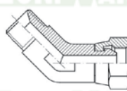
CODO 45° MACHO FIJO BSP 60° - HEMBRA LOCA BSP 60° RC6054
