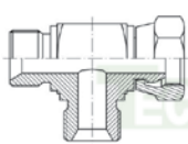
TE MACHOS FIJOS BSP 60° HEMBRA LOCA LATERAL BSP 60° RC6039
