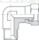
CODO 90° MACHO FIJO BSP 60° - HEMBRA LOCA BSP 60° RC6044
