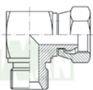
CODO 90° MACHO FIJO BSP 60° - HEMBRA LOCA RC6035
