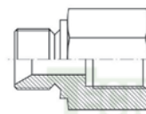
MACHO FIJO BSP 60° - HEMBRA FIJA BSP RC6017
