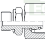
MACHO FIJO MÉTRICO, BSP PLANO - HEMBRA LOCA MÉTRICA CON JUNTA RCTN126MJ RCTN126BP
