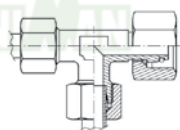
TE PARA TUBO - HEMBRA LOCA LATERAL RCTN121
