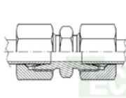
UNIÓN RECTA TUBO - TUBO SERIE LL - L - S RCTN098
