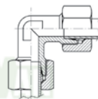
UNIÓN CODO TUBO - TUBO SERIE LL - L - S RCTN099
