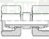
TUERCA LOCA - TUERCA LOCA METRICA CON JUNTA RCTN498
