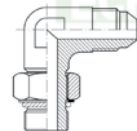
CODO 90° MACHO FIJO JIC 37° - MACHO BSP ORIENTABLE RC7018 en BSP PLANO RC7019 en UNF RC7048 en MÉTRICO
