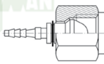
HEMBRA BSP CONO 60° RCMH1100
