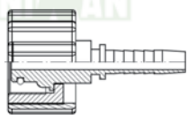
HEMBRA RCPR1221
